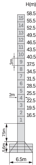
fixing underframe 底架固定式
